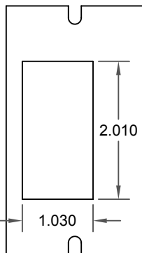
DP009 For Ortronics 2/TJ Bezel
